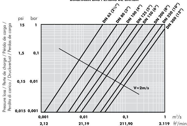
PRESSURE LOSS DIAGRAM DIAGRAMME DE PERTE DE CHARGE DIAGRAMA DE PÉRDIDAS DE CARGA DIAGRAMMA DELLE PERDITE DI CARICO DRUCKVERLUST-DIAGRAMM DIAGRAMA DAS PERDAS DE CARGA
